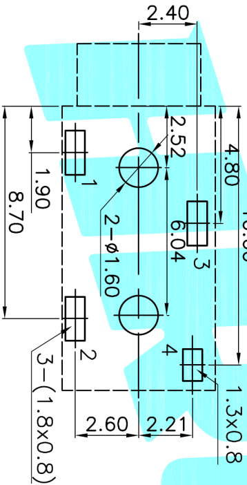
P.C.B LAYOUT(copper--sided view)
